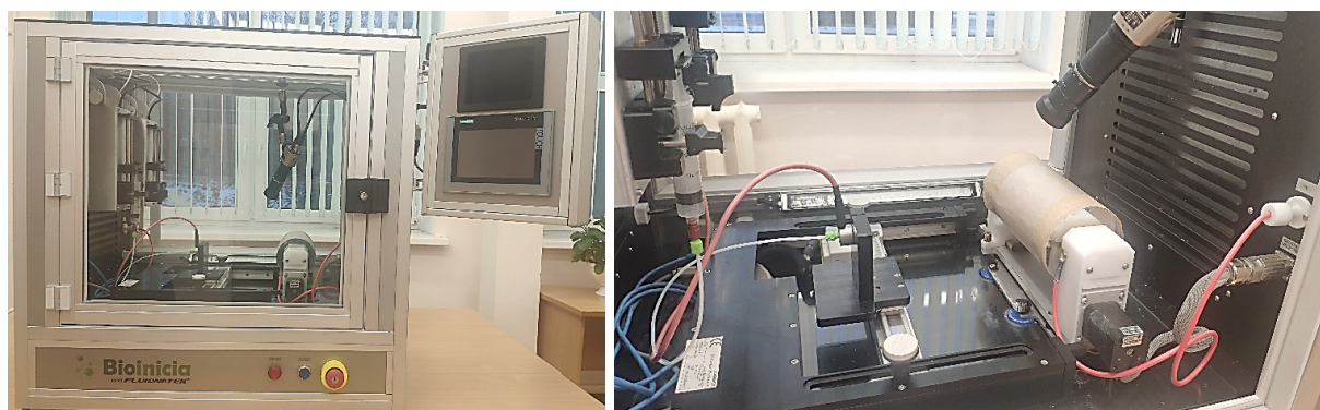
Рисунок 1 – Установка Fluidnatek LE-50 Figure 1 – Electrospinning machine Fluidnatek LE-50
