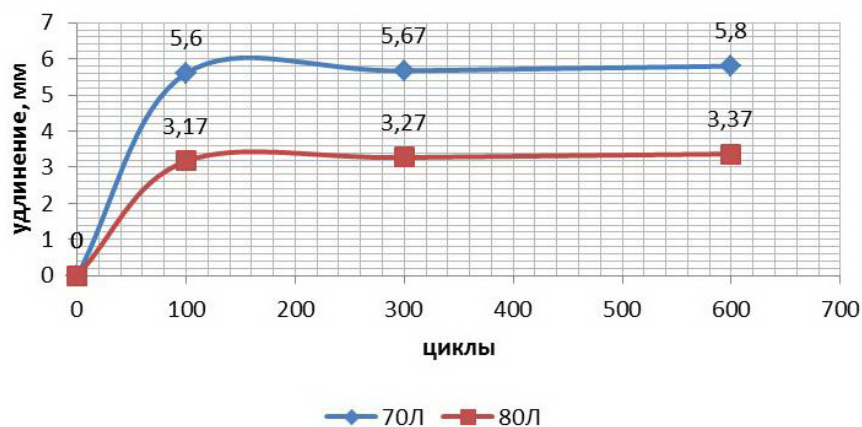
Рисунок 1 – График зависимости остаточной циклической деформации от числа циклов нагружения
