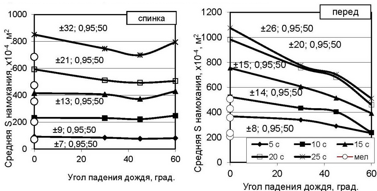
Рисунок 1 – Площадь намокания переда и спинки в процессе дождевания
