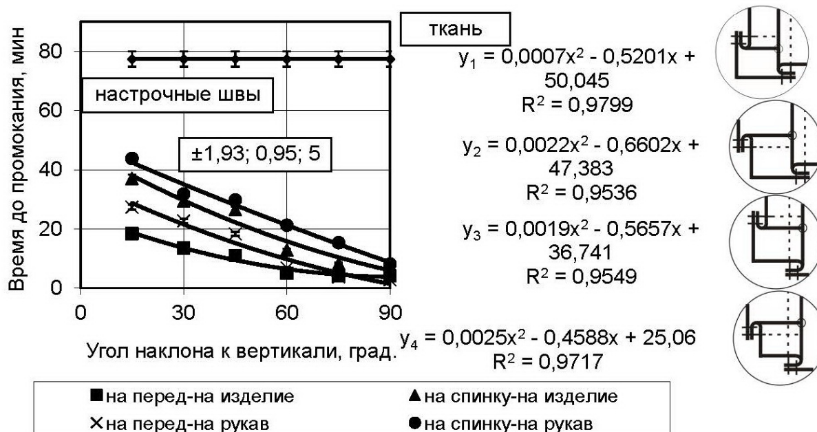
Рисунок 4 – Зависимость времени промокания плечевого узла изделия от угла воздействия воды и способа выполнения настрочных швов
