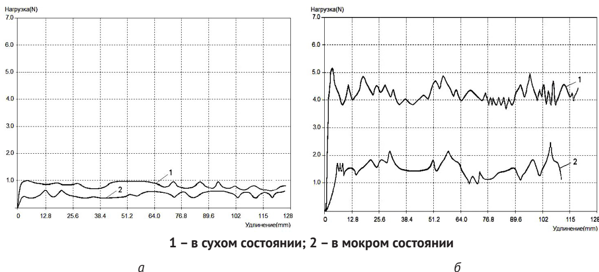
Рисунок 3 – Графики отслаивания отделочного покрытия от поверхности кожи арт. Нанпа: а – с естественной лицевой поверхностью; б – со шлифованной лицевой поверхностью
