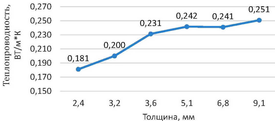
Рисунок 3 – Зависимость коэффициента теплопроводности силикона от толщины
