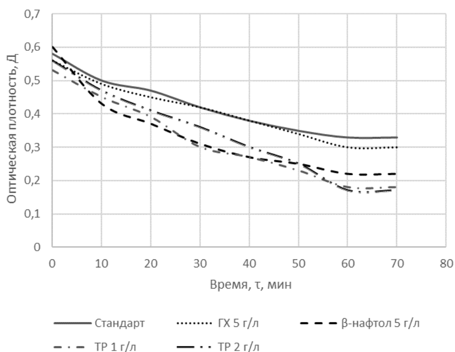
Рисунок 3 – Зависимость оптической плотности ( D ) от времени ( \tau ) крашения полиамидной ткани
