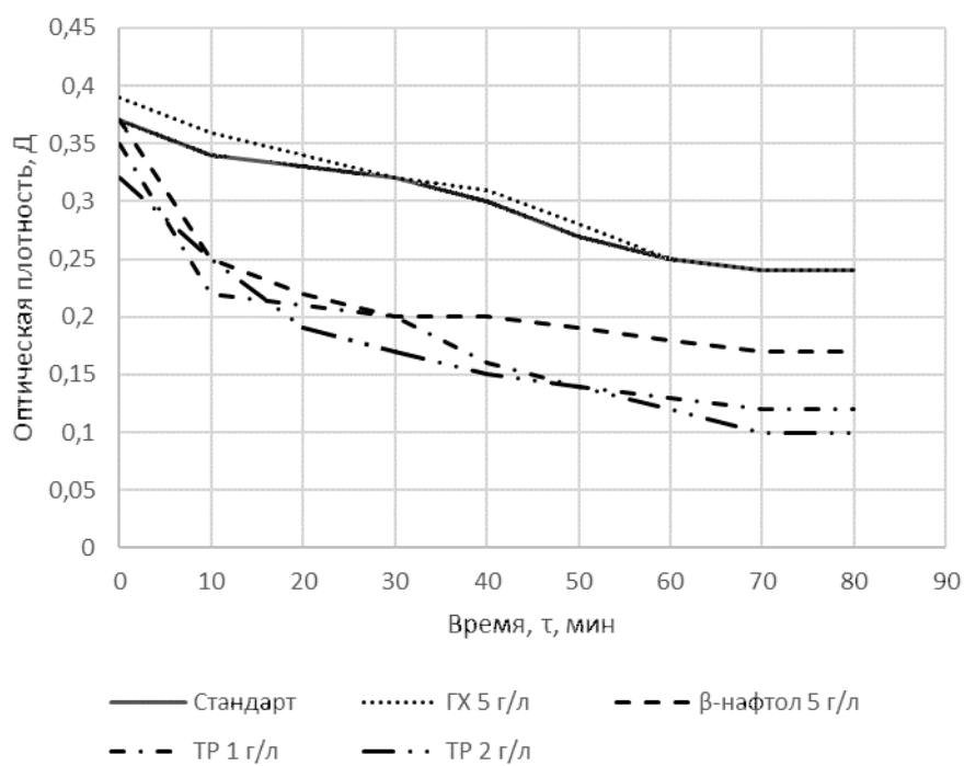
Рисунок 2 – Зависимости оптической плотности ( D ) от времени ( \tau ) крашения полиэфирной ткани
