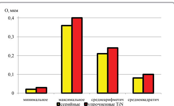
Рисунок 4 – Сравнительная диаграмма величины овальности шаров перед и после процесса нанесения слоя TiN
