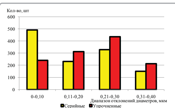
Рисунок 2 – Диаграмма частоты отклонения диаметров шаров от номинала перед и после процесса нанесения TiN
