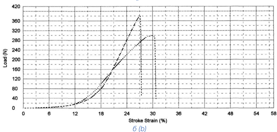
Рисунок 5 – Кривые прочности на разрыв по утку и основе:
