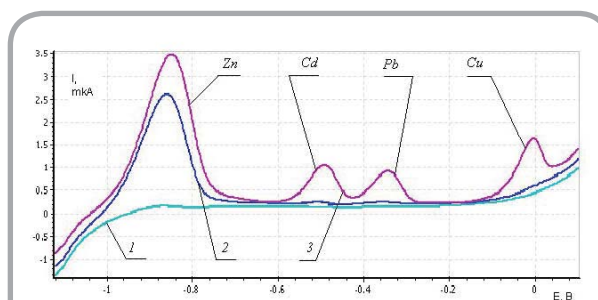
Рисунок 1 – Анодные вольтамперные кривые: 1 – фонового электролита (0,35 М водный раствор муравьиной кислоты); 2 – пробы образца экстракта дыма сигарет № 3 (KENT HD (4)); 3 – пробы образца экстракта дыма с добавкой стандартного раствора, содержащего по 2 мг/л Zn , Cd , Pb , Cu .
