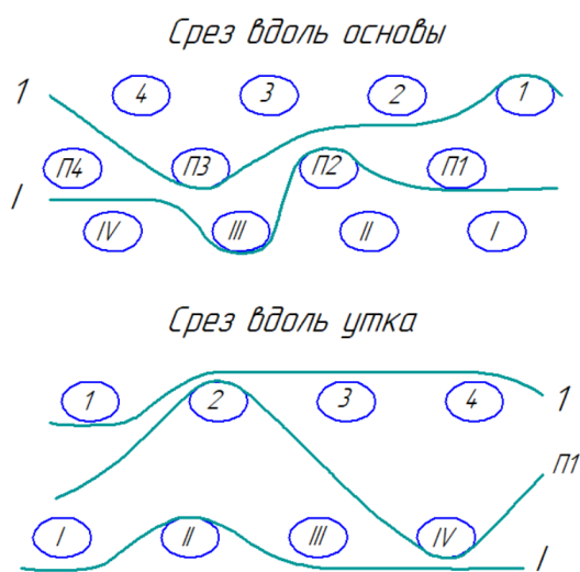
Рисунок 5 – Расположение нитей основы и утка в структуре двухслойной ткани с прижимными нитями утка Figure 5 – The arrangement of warp and weft threads in a two-layer fabric with pressed weft threads
