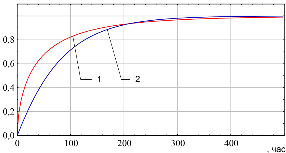
Рисунок 2 – Зависимость уровня накопления структурных повреждений ППН от времени воздействия УФ излучения: 1– нить BCF 260 текс (ф. Filartion); 2 – нить BCF 180 текс (ф. Aracta)
