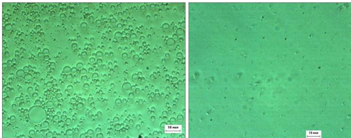
Рисунок 1 – Фазный состав эмульсола: а – 10% эмульсия на основе масла ВД-3, жирной кислоты и неанола; б – 10% эмульсия на основе нефтяного экстракта, жирной кислоты и неанола. Концентрат эмульсола подвергнут ультразвуковой обработке по разработанной методике
