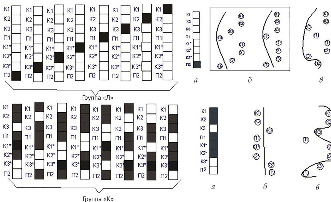
Рисунок 8 – Объединённая группа «К», «Л», графические изображения (а) и продольные разрезы (б, в) нитей смешанного гобелена
