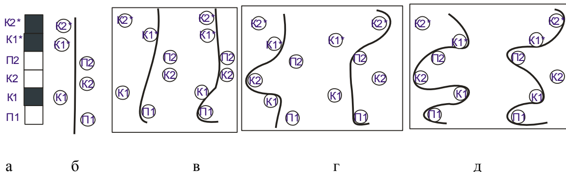
Рисунок 12 – Графическое изображение (а) переплетения нити основы, расположенной над нитями утка K1, K1*, K2*, и соответствующие ему продольные разрезы (б, в, г, д) в классическом основном гобелене для группы нитей «Ж»
