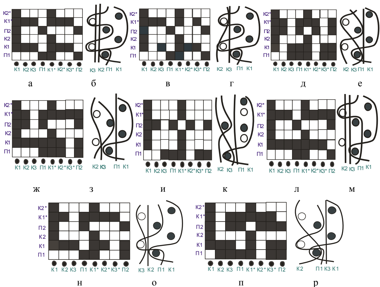
Рисунок 2 – Модельные переплетения VII (а), VIII (в), IX (д), X (ж), XI (и), XII (л), XIII (н), XIV (п), продольные разрезы (б, г, е, з, к, м, о, р) для полотняного эффекта классического гобелена
