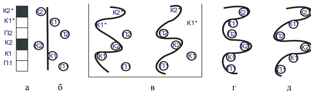
Рисунок 7 – Графическое изображение (а) переплетения нити основы, расположенной над нитями утка К2, К2*, и соответствующие ему продольные разрезы (б, в, г, д) в классическом основном гобелене для нитей группы «Б»
