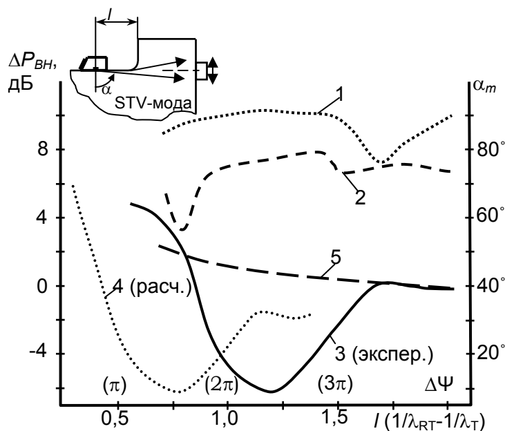
Рисунок 5 - Характерные изменения углов максимума \alpha_m амплитуды результирующей TV-моды (1, 2) и разницы максимумов \Delta P_{BH} = (P_B)_{max} - (P_H)_{max} (3, 4) в зависимости от расстояния до выступа: 1 - \alpha_m для (P_B)_{max} , 2 - для (P_H)_{max} ; 5 - \Delta P_{BH} = (P_H)_{max} - (P_{AT})_{max} в отсутствие выступа
