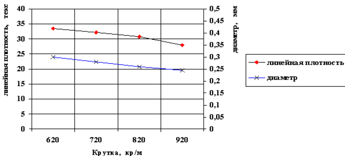
Рисунок 7 – Зависимость линейной плотности и диаметра высокоэластичной пряжи пневмомеханического способа прядения от крутки
