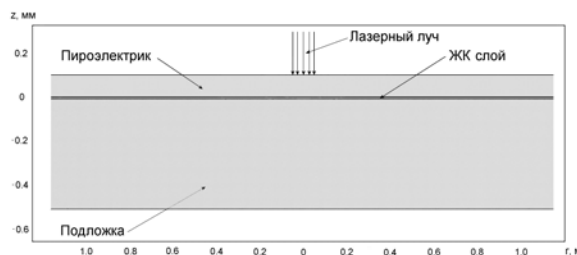
Рисунок 1 - Схематичное изображение структуры преобразователя изображения
