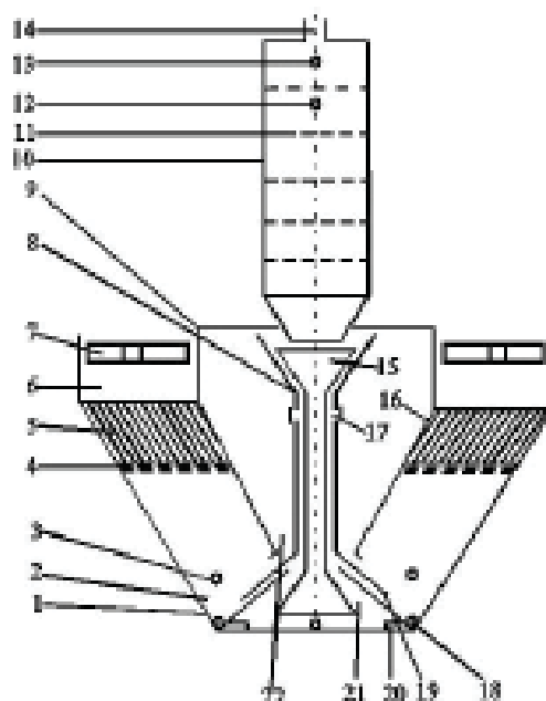
Рисунок 1 – Схема блока биохимической очистки: 1 – корпус; 2 – зона зависшего слоя; 3 – выпуск циркулирующего активного ила; 4 – сетка-электрод; 5 – ляминаторы; 6 – защитная зона; 7 – сборные лотки, выход очищенной воды; 8 – перегородка; 9 – перекрытие; 10 – корпус аппарата с пенными слоями; 11 – тарелки; 12 – впуск циркулирующего ила; 13 – впуск сточной воды; 14 – выпуск воздуха; 15 – направляющая колонка; 16 – перегородка; 17 – переливные окна с шиберами; 18 – система выпуска; 19 – «зубы»; 20 – аэраторы; 21 – зона аэрации; 22 – зона дегазации
