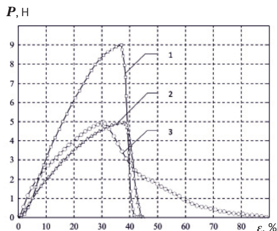
Рисунок 2 – Диаграмма растяжения «нагрузка – относительное удлинение» ПП нитей различного способа получения: 1 – Humь Frize «Tattekstil» (Турция); 2 – Humь Heat-Set «Arasta» (Турция); 3 – Humь BCF «Filarlois» (Франция)
