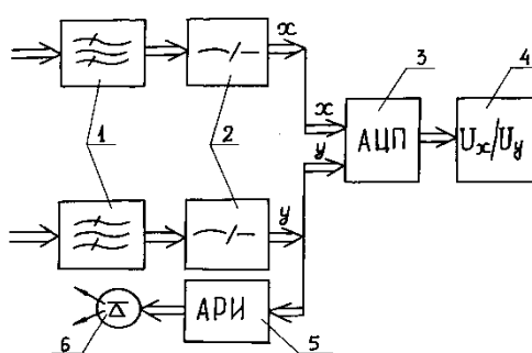
Рисунок 3 - Принципиальная схема блока питания и обработки сигналов
